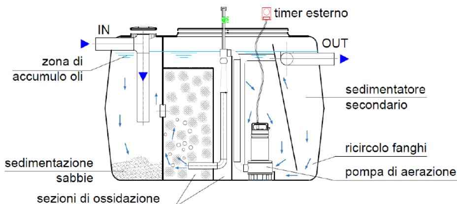
Figura n. 9 - Particolare costruttivo (sezione) del sistema di trattamento fisico-biologico delle acque di lavaggio
