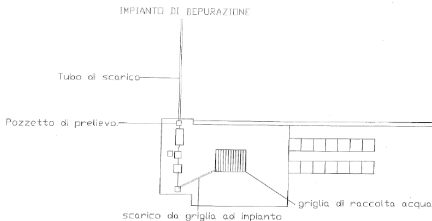
Figura n. 10 - Layout in pianta dell'impianto di depurazione fisico-biologico
