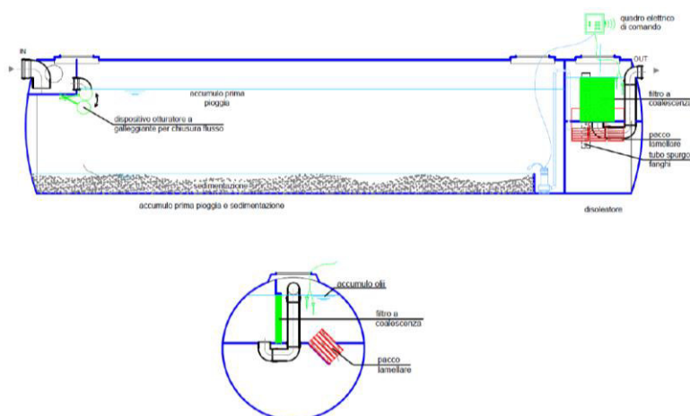
Figura 11 - Particolari costruttivi e sezione dell'impianto di trattamento delle acque di prima pioggia
